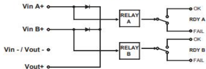
Diagrama de Circuito
